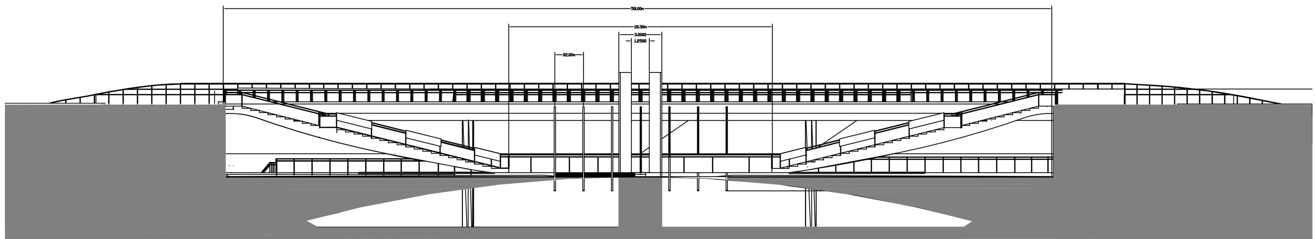
مقطع A-A ۱:۲۰۰
